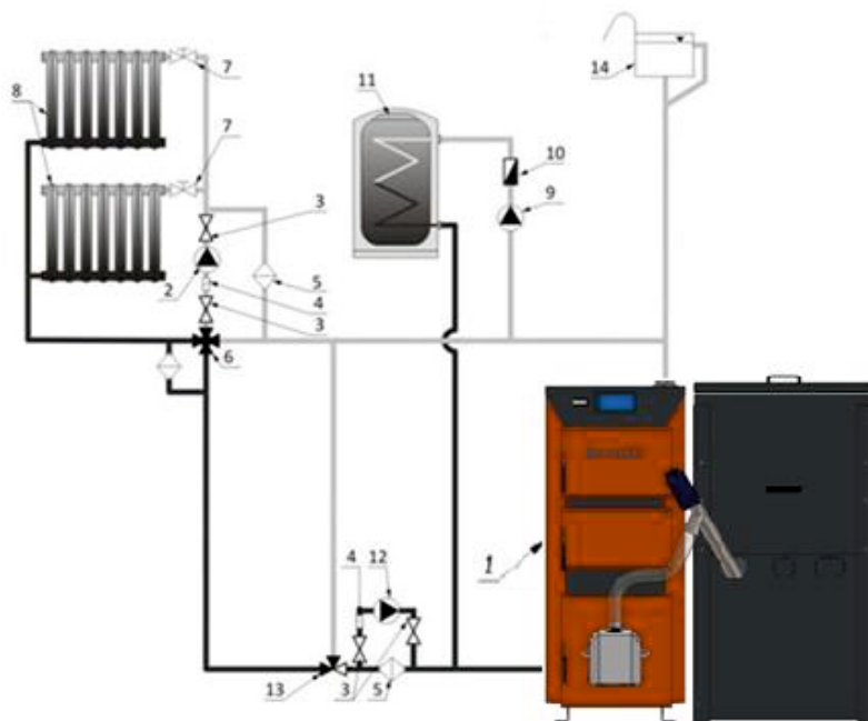
Rys. 10 Przykładowy schemat instalacji grzewczej systemu otwartego
