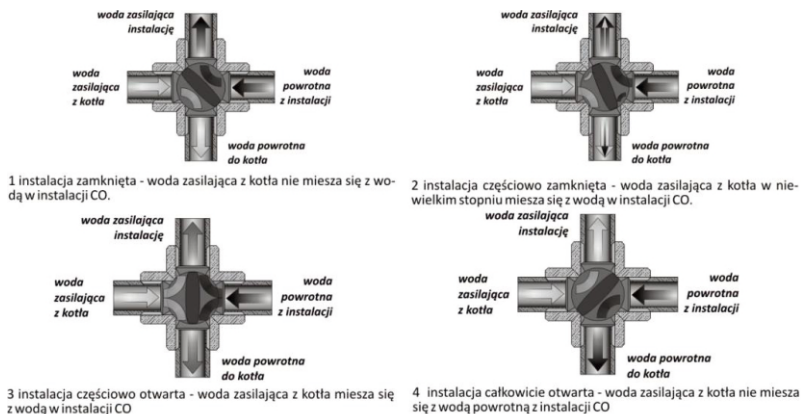
Rys. 9 Zasada działania zaworu czterodrogowego
