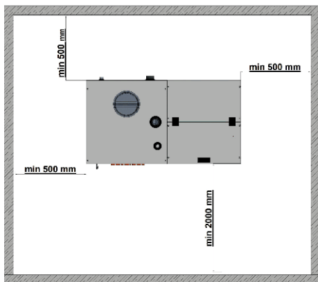
Rys. 3 Ustawienie kotła w pomieszczeniu kotłowni
