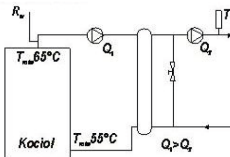
Rys. 8 Schemat połączenia kotła z instalacją grzewczą z wykorzystaniem sprężła wodnego.
