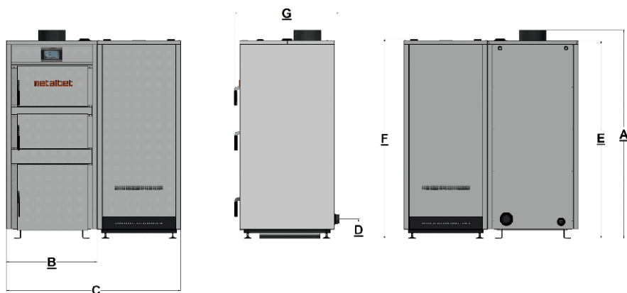
Rys. 2 Podstawowe wymiary kotłów AQUA ECO PELLET 10-25 kW z osprzętem( patrz tab. nr 3 )
