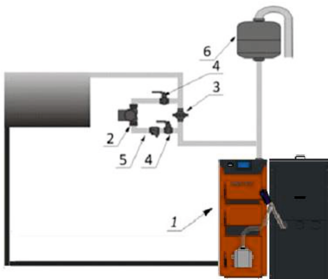
Rys. 5 Wykonanie obejścia grawitacyjnego
