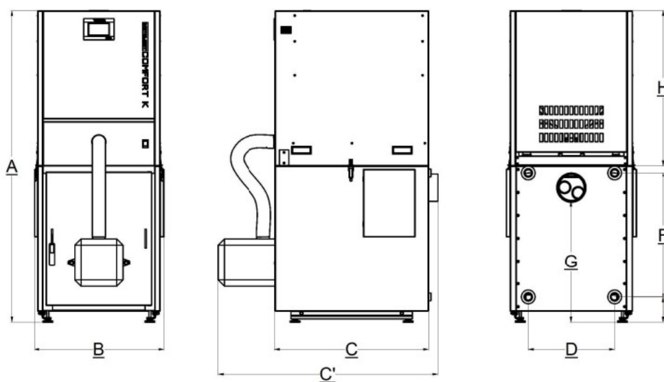
Rys. 3. Podstawowe wymiary kotła Comfort KS
