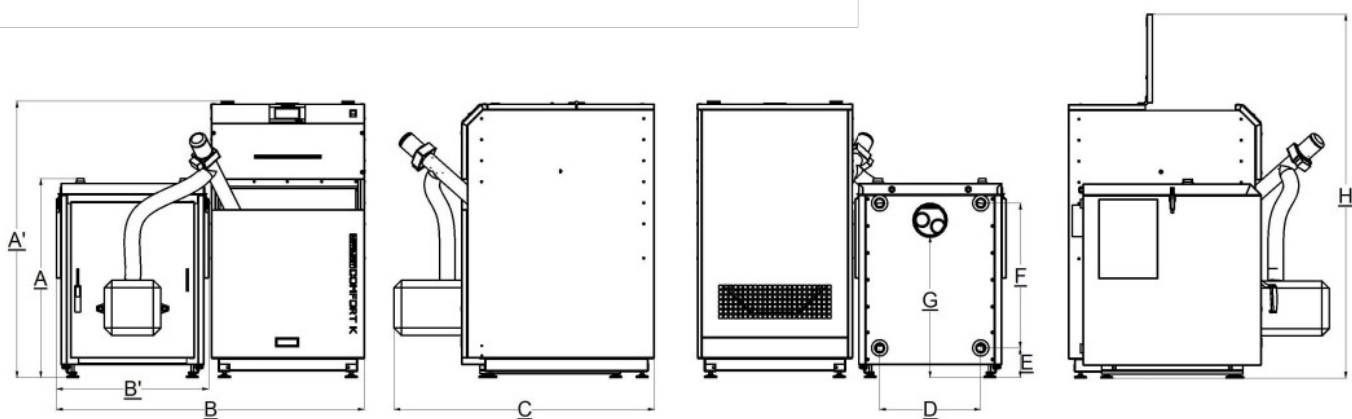
Rys. 1a. Schemat kotła Comfort KS z zasobnikiem z prawej lub z lewej strony
