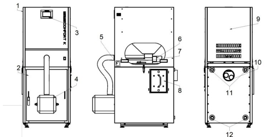
Rys. 1. Schemat kotła Comfort KS z zasobnikiem górnym
