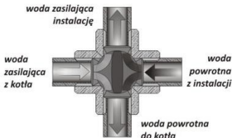
Rys. 9 Zasada działania zaworu czterodrogowego
