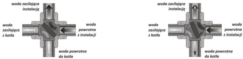
Rys. 8 Schemat połączenia kotła z instalacją grzewczą z wykorzystaniem sprzęgła wodnego.
