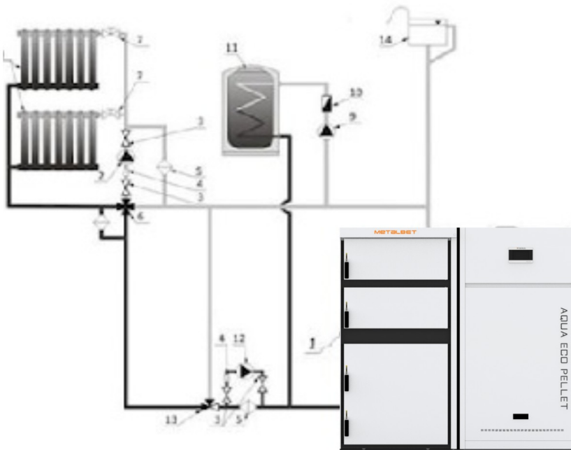
Rys. 10 Przykładowy schemat instalacji grzewczej systemu otwartego
